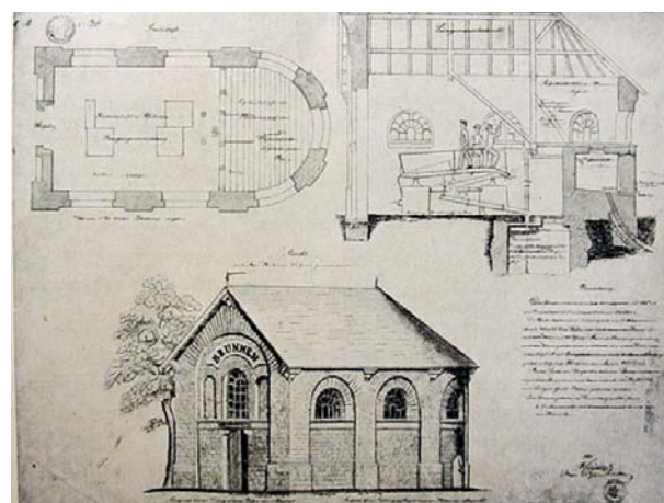
Zeichnung des Brunnenhauses der königlich preussischen Genie Direktion (AnLux)
